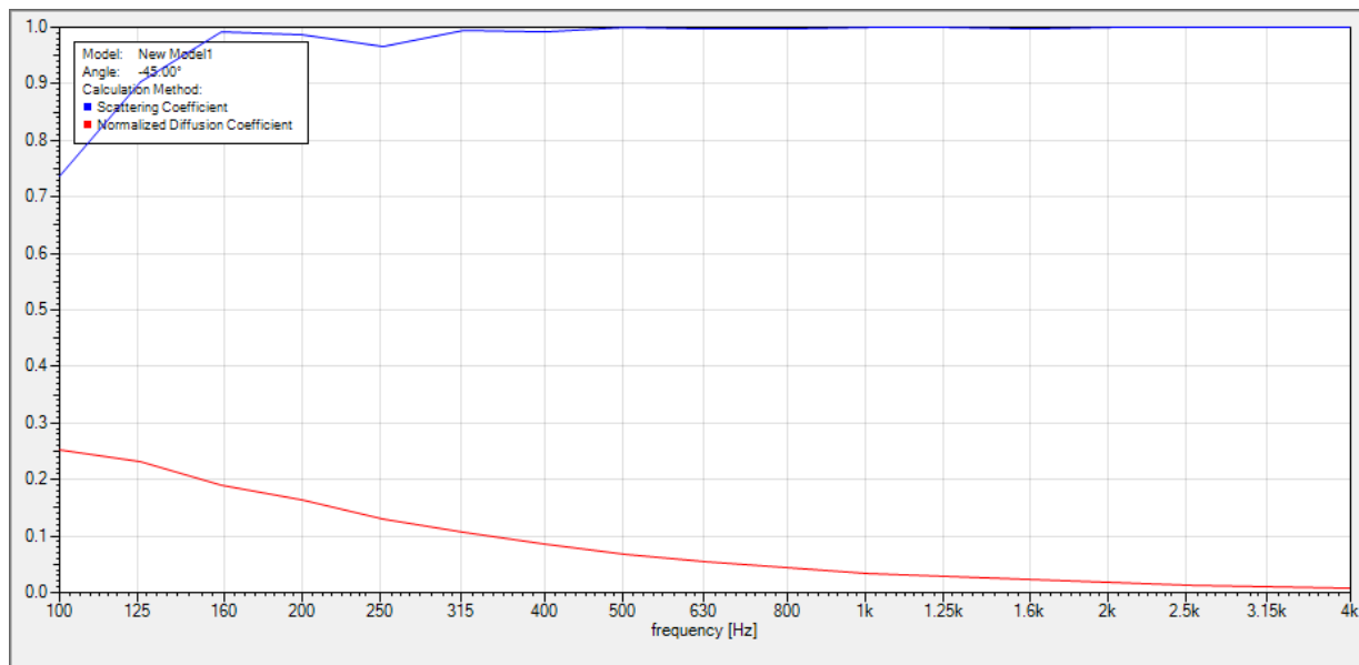
ISO 17497-2 Diffusion & Scattering Test Data
