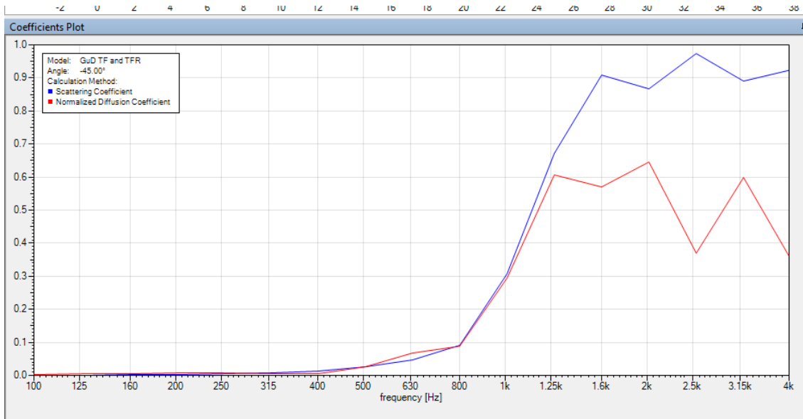
ISO 17497-2 Diffusion & Scattering Test Data
